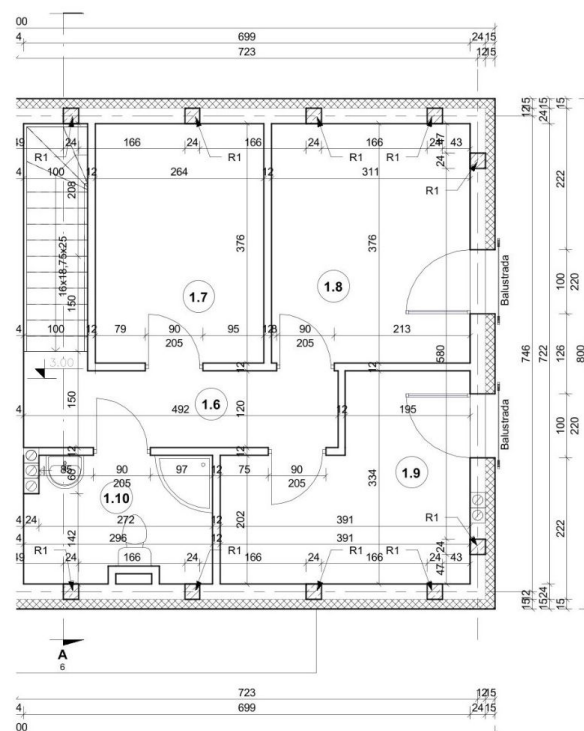
Rzut poddasza
