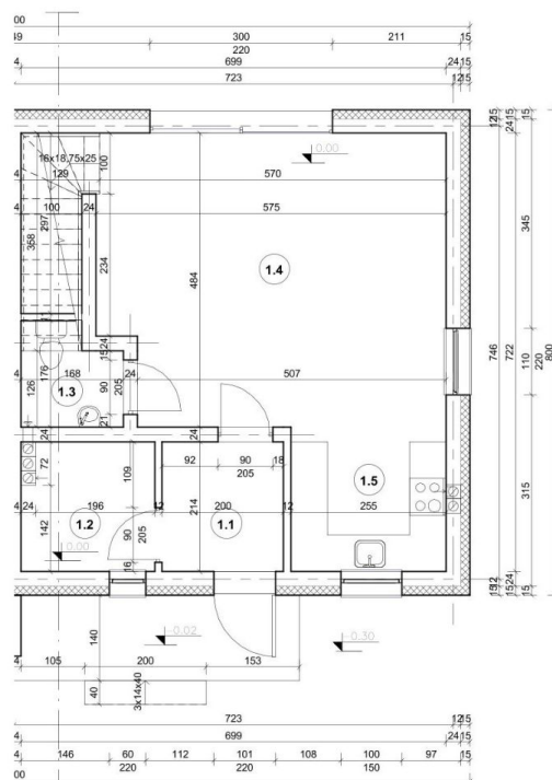
Rzut parteru
