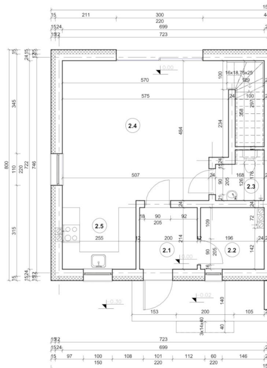
Rzut parteru
