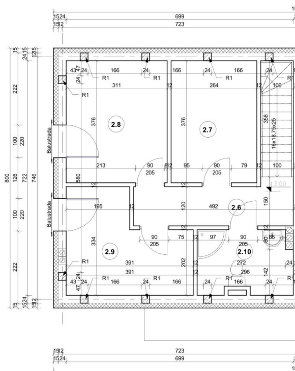
Rzut poddasza
